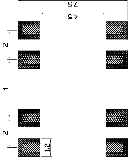
安装图 (PCB LAYOUT PLAN)
